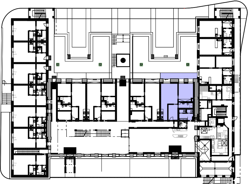
Schéma půdorys
